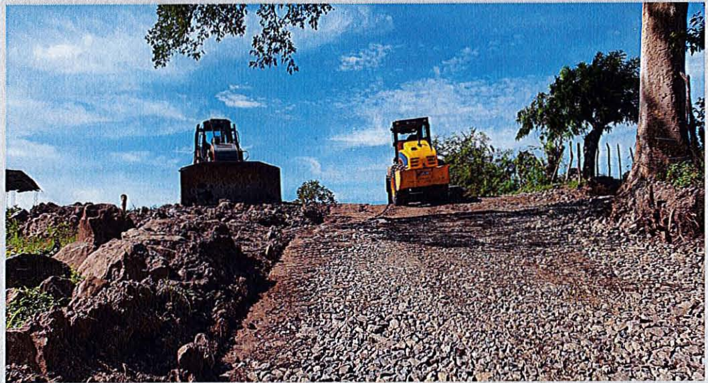
Foto 4: Reconstrucción de la calle de acceso de la comunidad Guajoyito.
